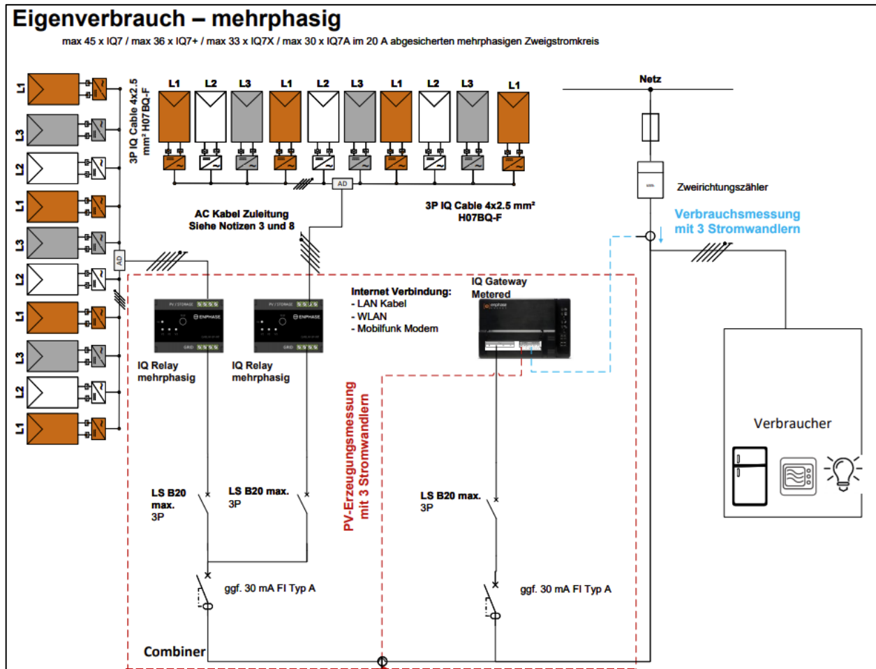
Abbildung 3 Konfiguration Nr. 3:2 x 3-phasiger PV, Kein Speicher
