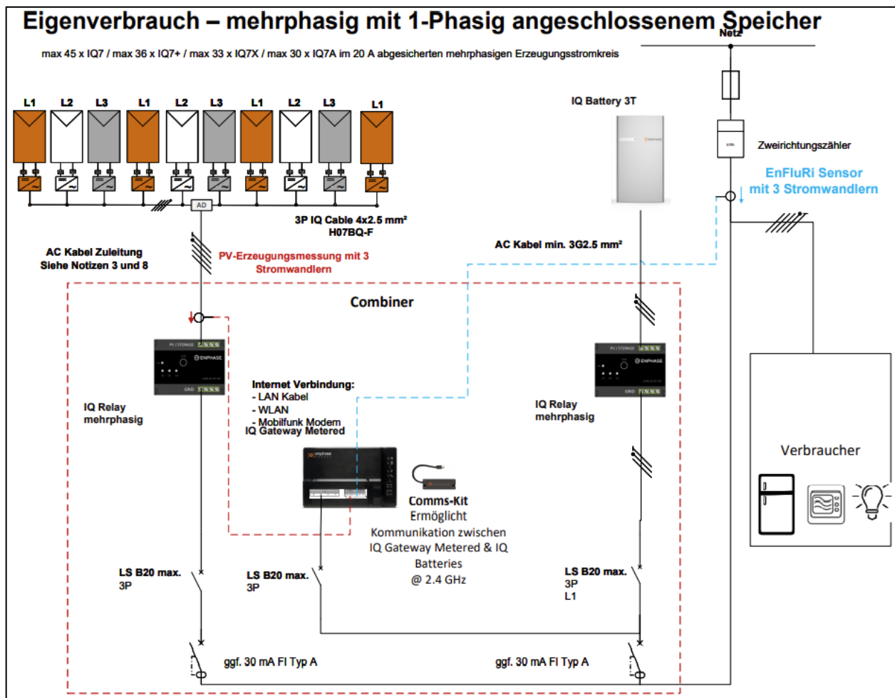
Abbildung 6 Konfiguration Nr. 6: 1 x 3P PV, 1 x IQ Batterie 3T
