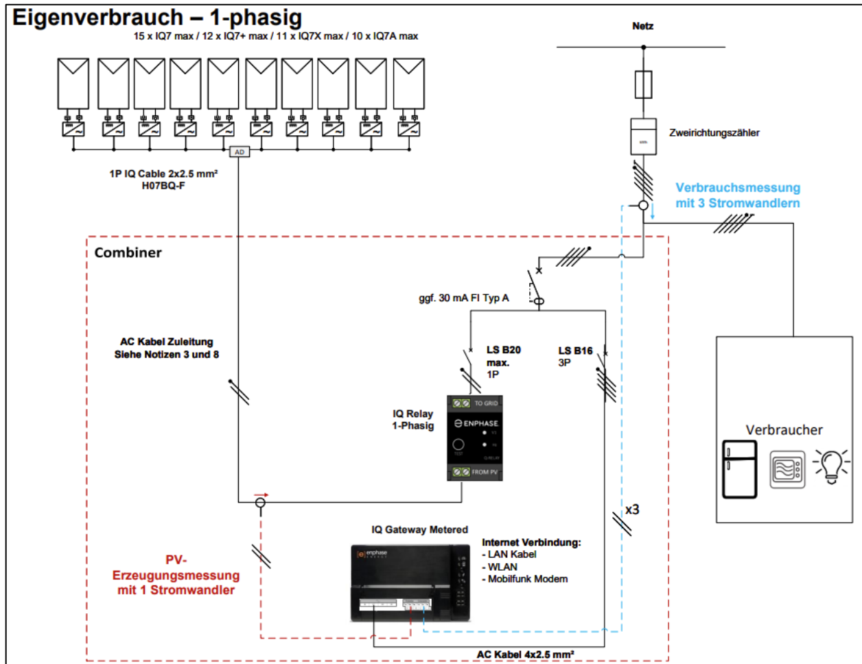
Abbildung 1 Konfiguration Nr. 1 (Nur PV): 1 x 1-phasiger PV, Kein Speicher
