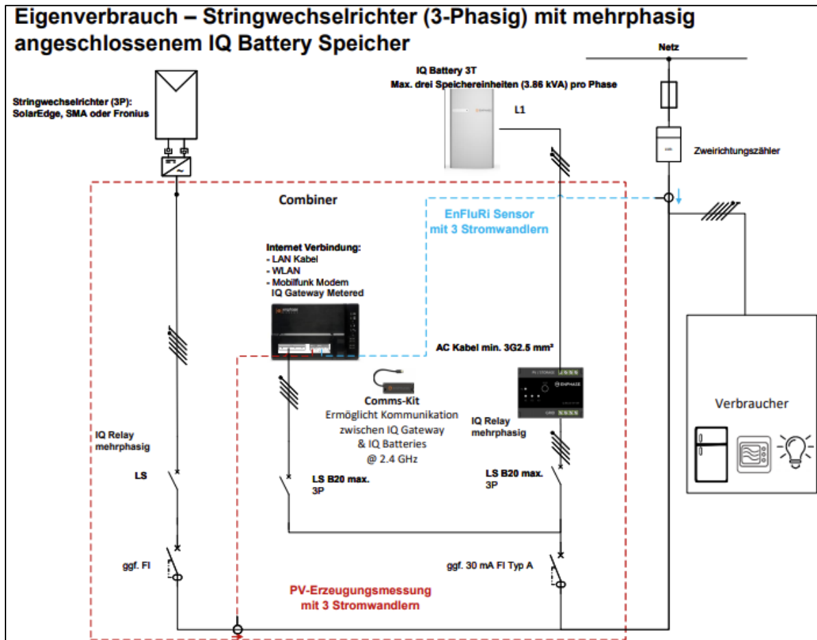
Abbildung 10 Konfiguration Nr. 10: 1 x String-Wechselrichter PV, 1 x IQ Batterie 3T
