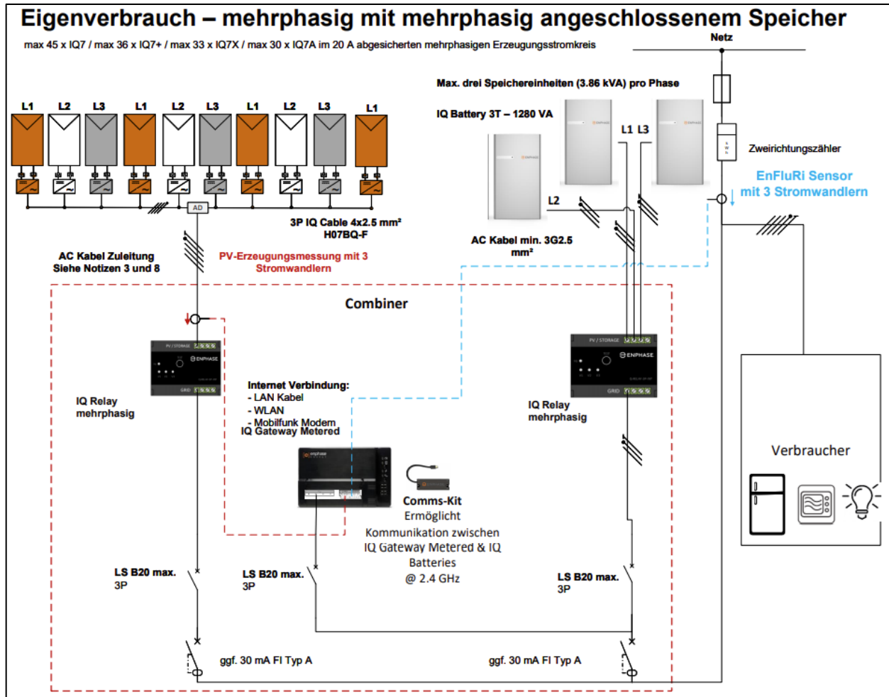
Abbildung 8 Konfiguration Nr. 8: 1 x 3P PV, 3 x IQ Batterie 3T
