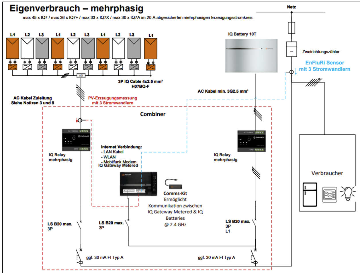
Abbildung 4 Konfiguration Nr. 4: 1 x 3P PV, 1 x IQ Batterie 10T
