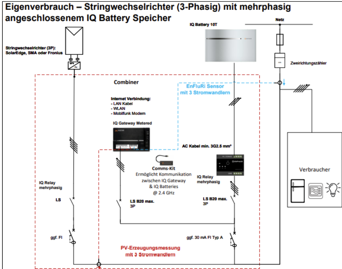
Abbildung 9 Konfiguration Nr. 9:1 x String-Wechselrichter PV, 1 x IQ Batterie 10T
