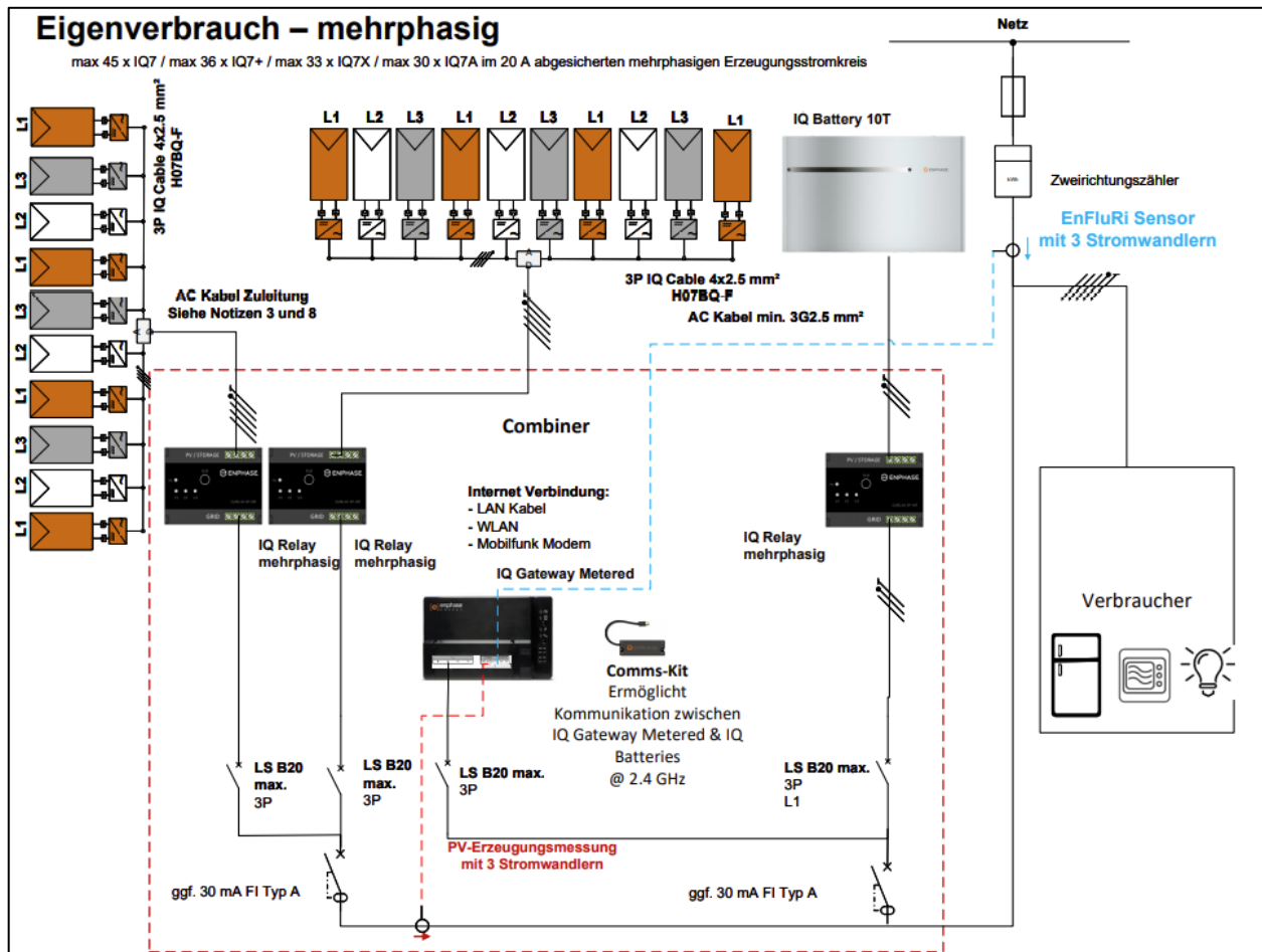
Abbildung 5 Konfiguration Nr. 5: 2 x 3P PV, 1 x IQ Batterie 10T
