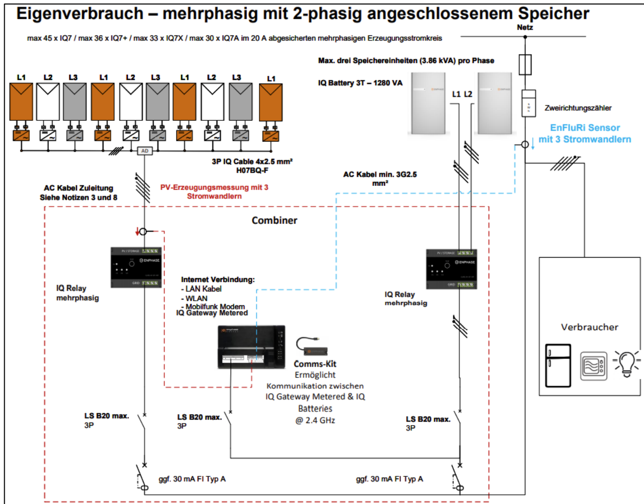
Abbildung 7 Konfiguration Nr. 7: 1 x 3P PV, 2 x IQ Batterie 3T
